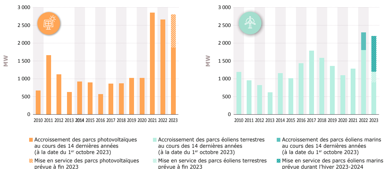
Figure 5 Évolution des parcs éolien et photovoltaïque
