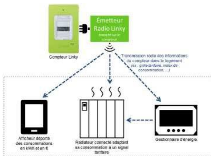
Figure 2 Exemples d'utilisation de l'ERL – Source Enedis
