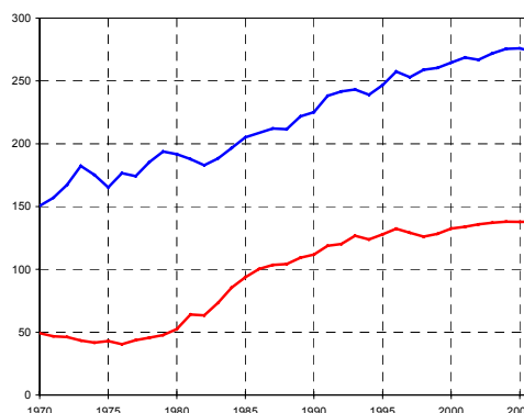
Fig. 7 : Production et consommation d'énergie primaire, non corrigées du climat (en Mtep).
