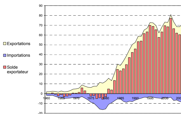
Fig. 5 : Commerce extérieur d'électricité depuis 1960 (en TWh).
