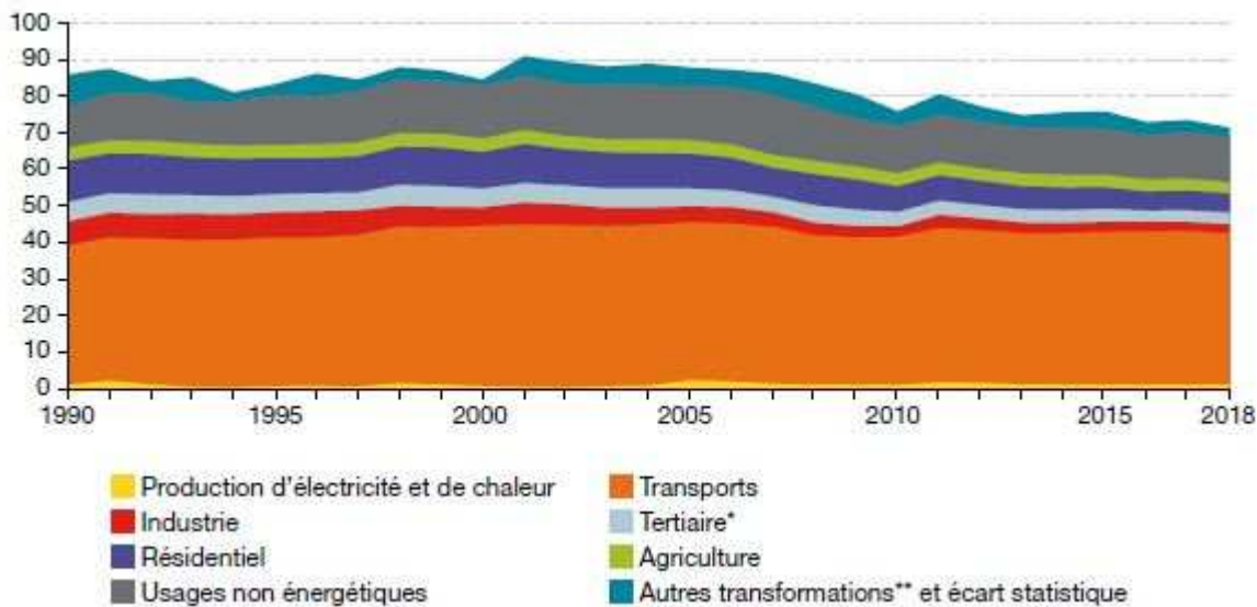
Figure 41 : Consommation primaire de produits pétroliers (hors biocarburants, soutes maritimes et aériennes internationales) en Mtep 42
