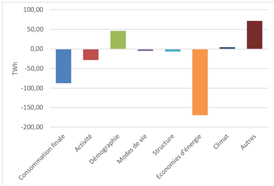
Figure 5. Décomposition de l'évolution de la consommation énergétique finale de la France entre 2006 et 2016 (en Mtep) (source : Odyssee, 2019)
