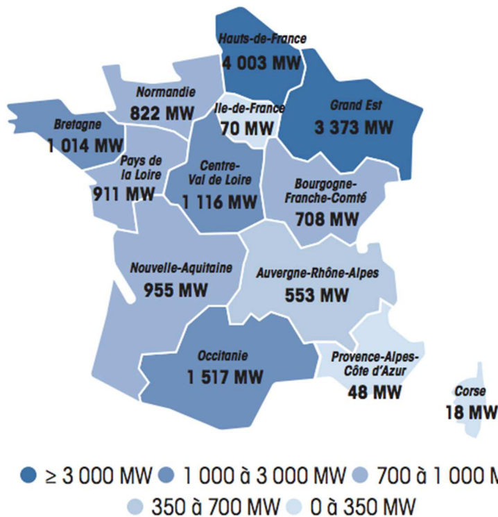
Figure 44 : Répartition régionale des capacités de production éolienne raccordées au 31 décembre 2018 (MW) (Source : RTE)
