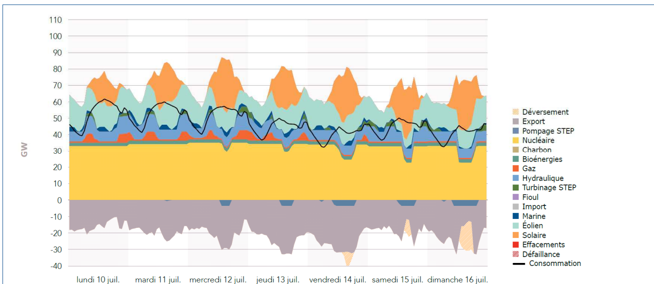
Figure 65 : Illustration de la production, de la consommation et des exportations sur une semaine estivale en 2035 (scénario Ampère) - Source : RTE, 2017
