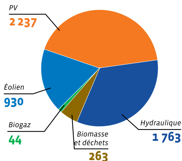
Répartition du parc EnR électrique régional au 30/09/18 (en MW)
