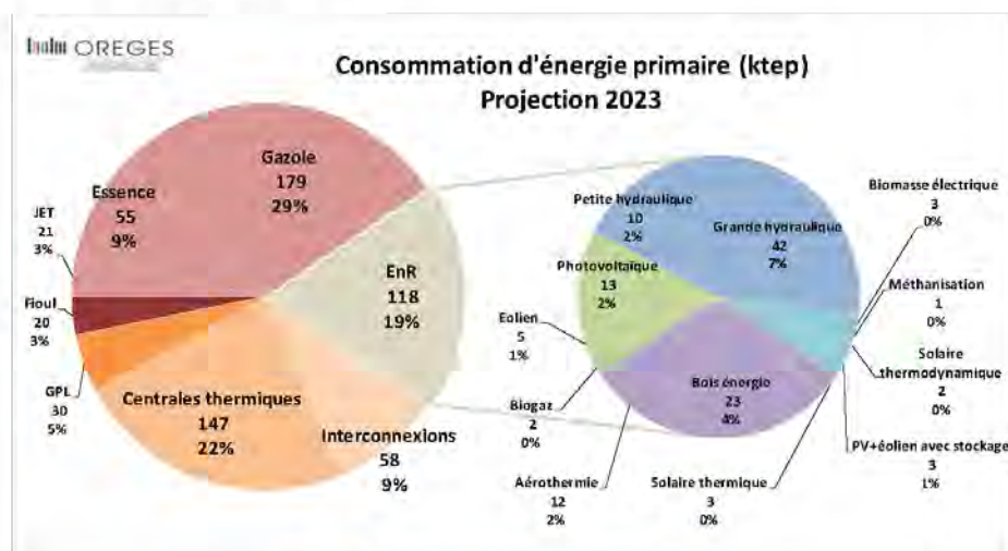
Figure 31 : Projection bilan énergie primaire en 2023
