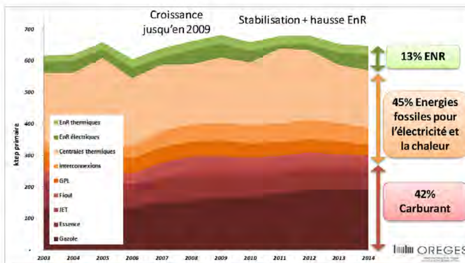
Figure 12 Evolution de la consommation d'énergies primaires de 2003 à 2014 (Sources OREGES de Corse)
