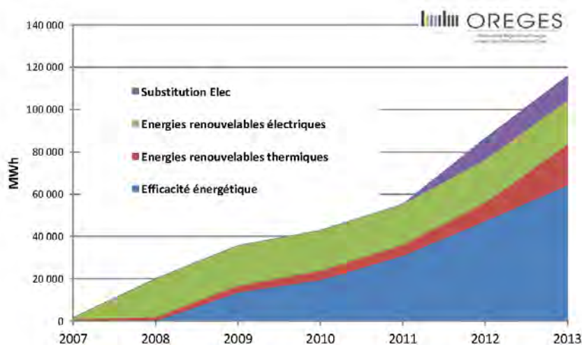
Figure 19 Bilan énergétique du Plan EnR-MDE 2007-2013 (Source OREGES de Corse)
