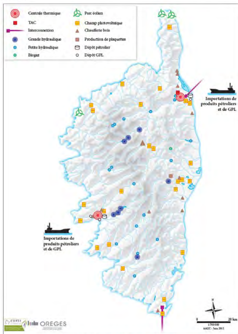
Figure 1 Système énergétique de la Corse - 2014 (Source OREGES de Corse)
