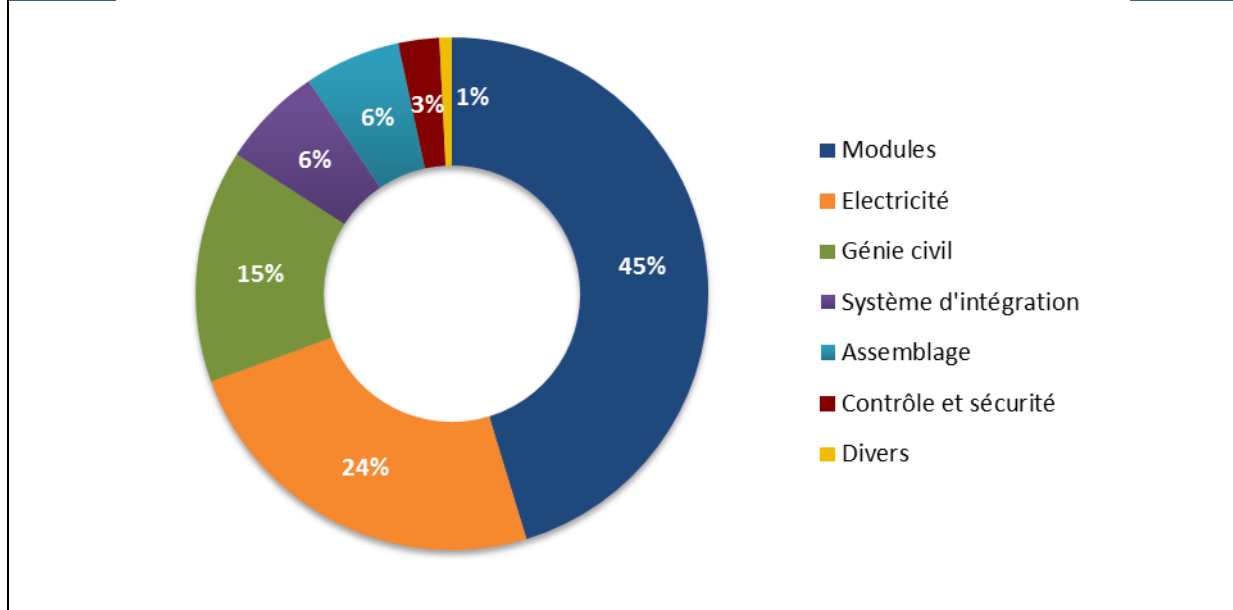
Figure 23. Ventilation moyenne des coûts d'installation de la centrale photovoltaïque
