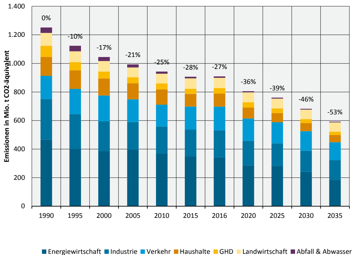
Abbildung 3-3-2: Entwicklung der gesamten Treibhausgasemissionen 1990 bis 2035 nach Quellbereichen im Mit-Weiteren-Maßnahmen-Szenario
