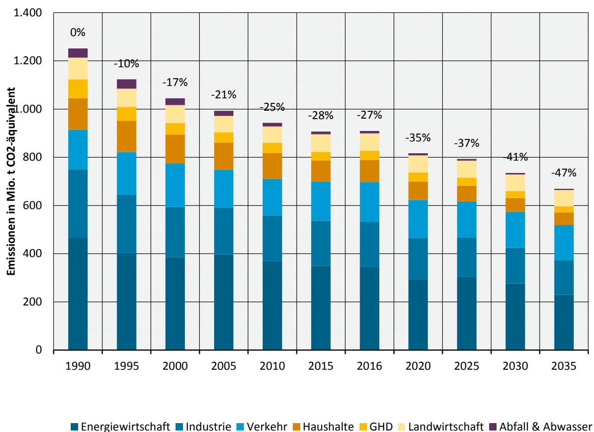
Abbildung 3-3-1: Entwicklung der gesamten Treibhausgasemissionen 1990 bis 2035 nach Quellbereichen im Mit-Maßnahmen-Szenario
