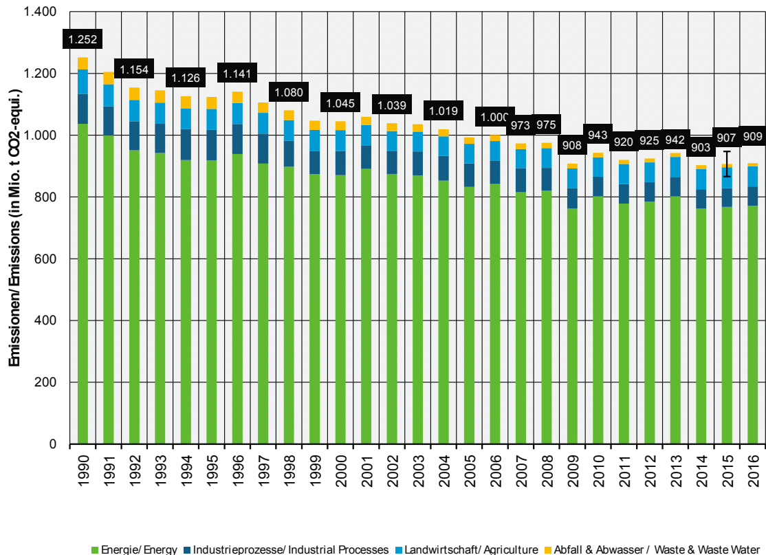
Abbildung 2: Emissionsentwicklung in Deutschland seit 1990, nach Kategorien
