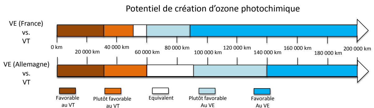
Figure 1-20 : Domaines de pertinence environnementale du véhicule électrique (France et Allemagne) comparés au véhicule thermique pour le potentiel de création d'ozone photochimique en 2012
