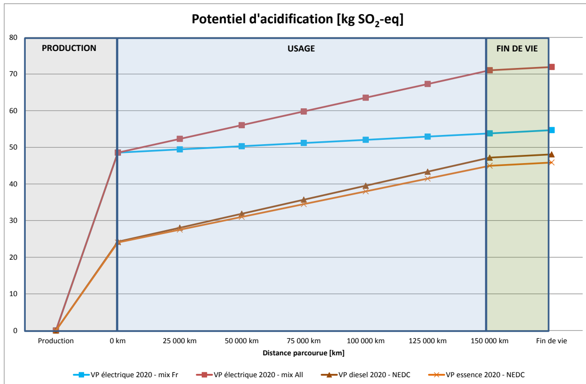
Figure 1-12 : Potentiel d'acidification pour les véhicules électriques français et allemand et les véhicules thermiques essence et diesel à l'horizon 2020 selon le scénario de référence
