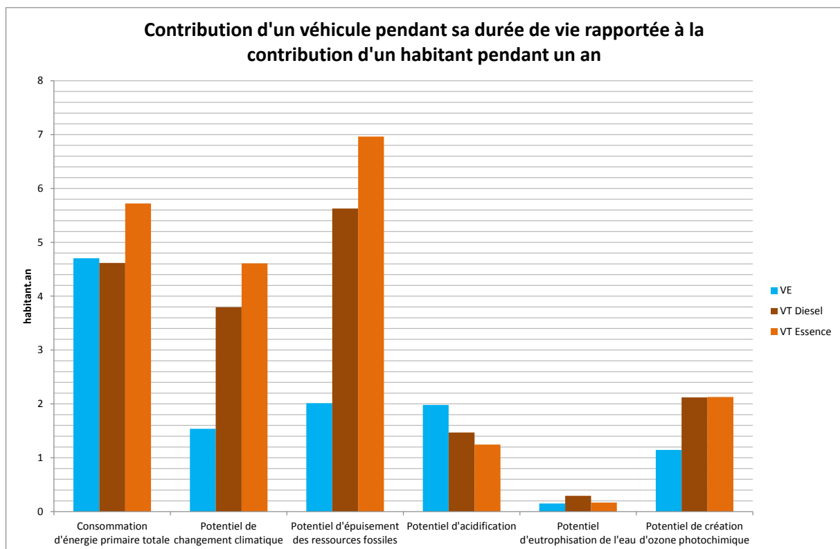
Figure 1-22 : Normation des six impacts potentiels retenus pour le VP en France en 2012
